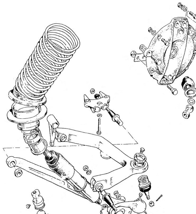
Schéma amortisseur long
