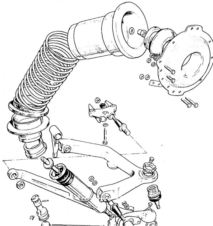
Schéma amortisseur court avec vérin
